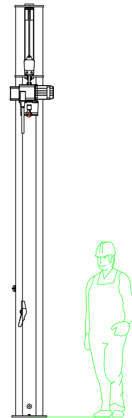
Ansicht A
