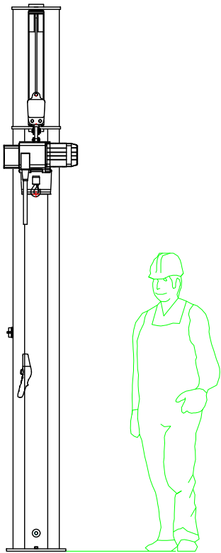
Ansicht A
