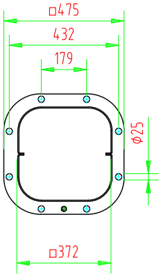
Lochbild 1:20
