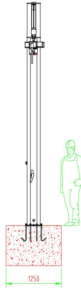
Ansicht A
