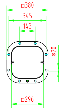
Lochbild 1:20
