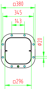
Lochbild 1:20
