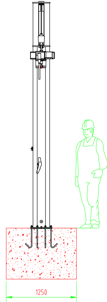
Ansicht A
