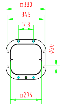
Lochbild 1:20
