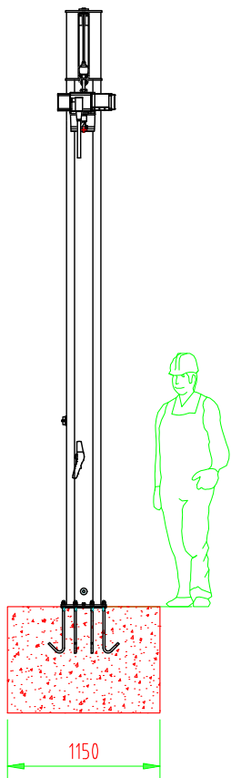
Ansicht A
