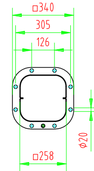
Lochbild 1:20
