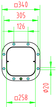
Lochbild 1:20
