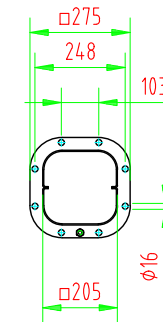
Lochbild 1:20
