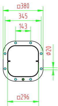
Lochbild 1:20
