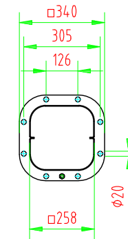
Lochbild 1:20
