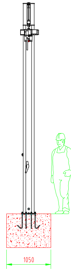
Ansicht A
