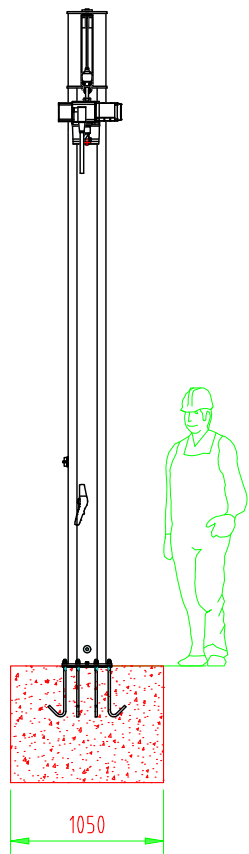
Ansicht A
