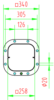
Lochbild 1:20
