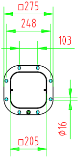
Lochbild 1:20
