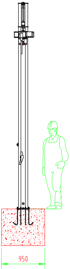
Ansicht A
