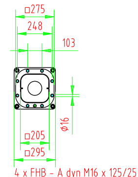
Lochbild 1:25
