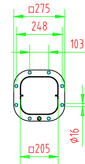
Lochbild 1:20
