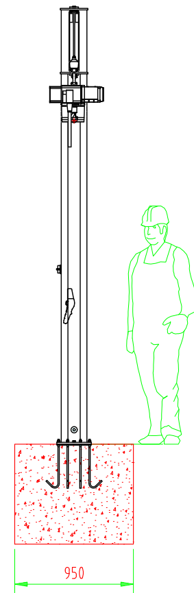
Ansicht A
