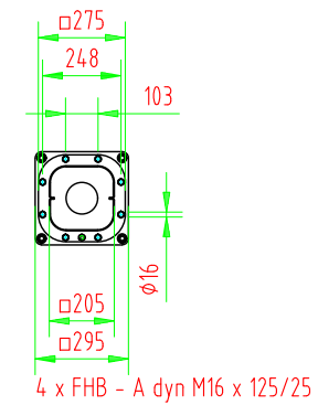
Lochbild 1:25
