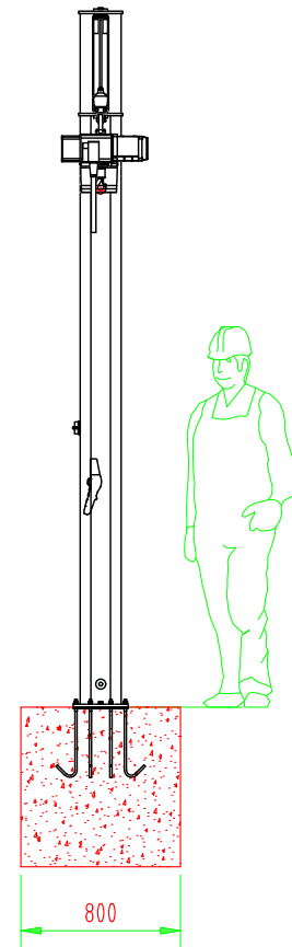
Ansicht A
